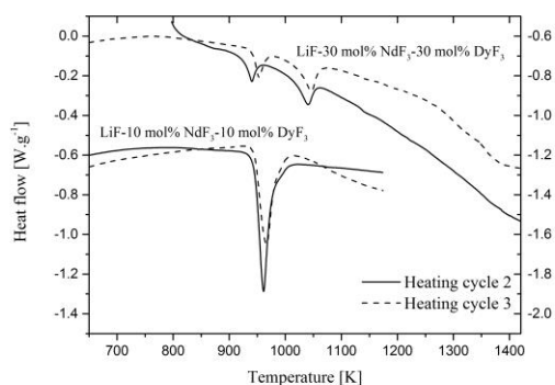
(b) LiF-DyF 3 -NdF 3
