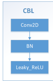
Fig. 5. Module CBL
