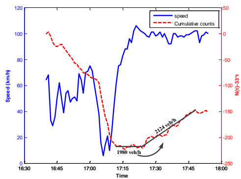
(d) Center lane, location 1, 28 May 2009
