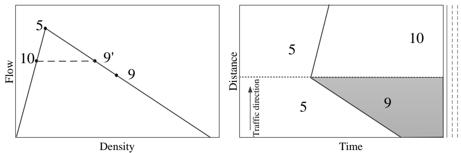
(d) Case 4: on-ramp node scenario
