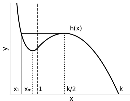
Fig. 20. The function h(x) .
