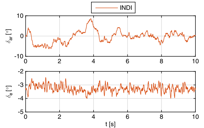
Fig. 27 Control inputs using INDI.
