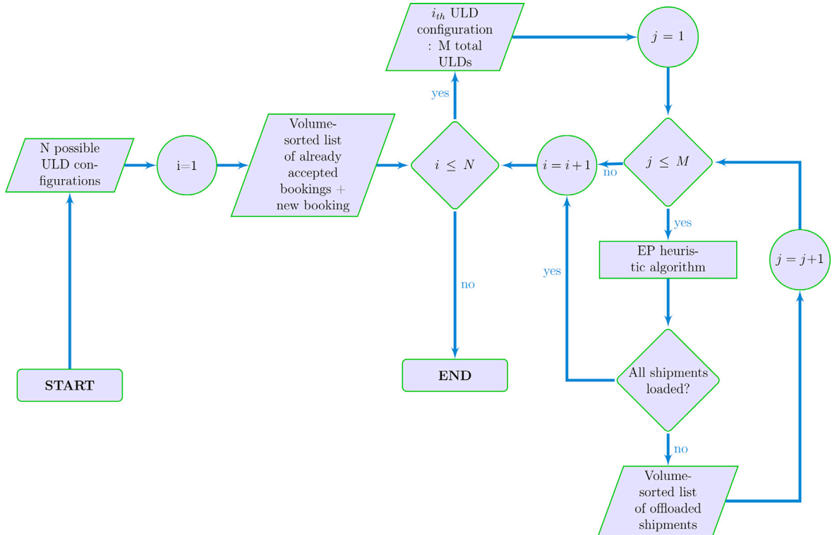
Fig. 14. 3D-MHKP model.
