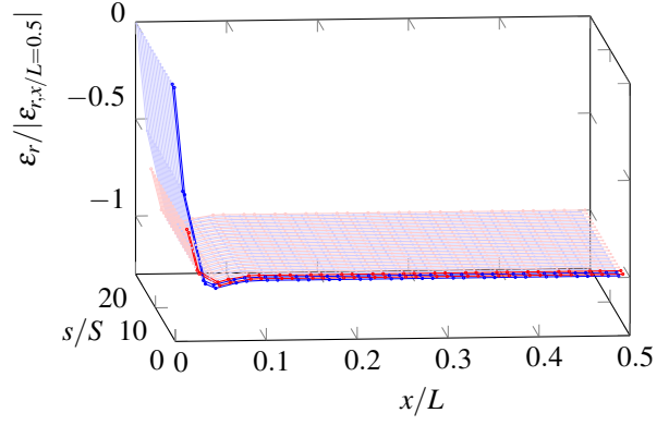
(d) (20,0) zigzag
