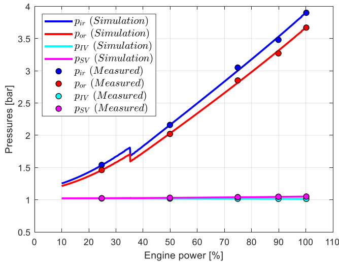
Fig. 12. Buchi pressures.
