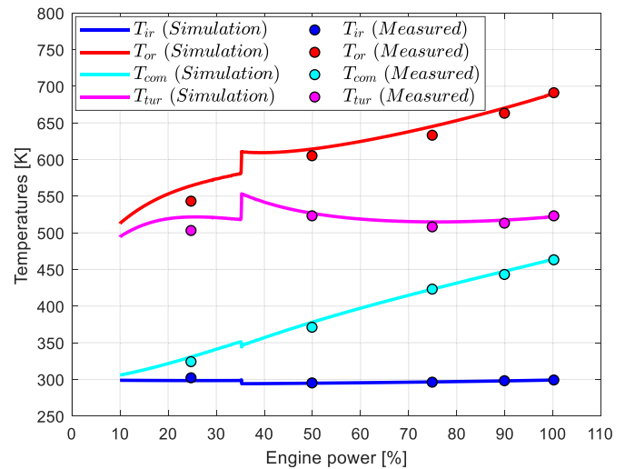
Fig. 11. Buchi temperatures.
