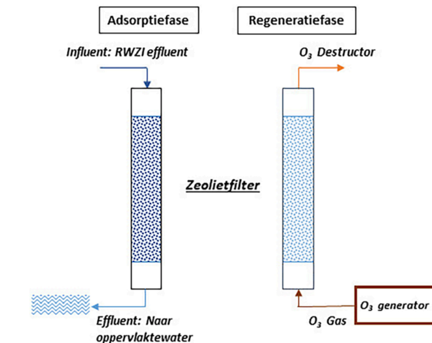
Het principe van AdOx: adsorptie van OMV's in een zeolietfilter, en regeneratie van een verzadigd zeolietfilter met ozongas.
