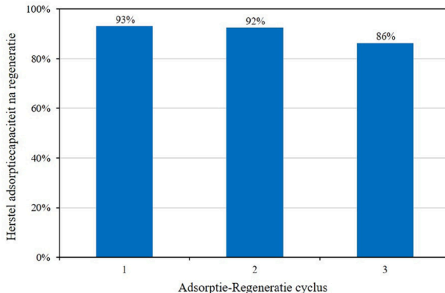
Adsorptiecapaciteit van een zeolietfilter voor acetaminophen (ACE) gedurende drie opeenvolgende adsorptie-regeneratie cycli.
