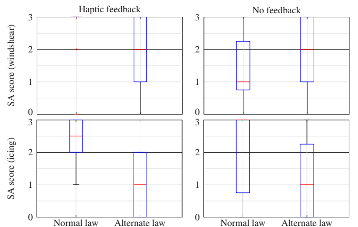
Fig. 12. SA scores for both scenarios.
