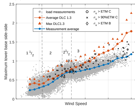
(d) Maximum Tower base side-side moment
