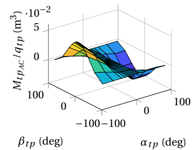
(d) Pitch moment coefficient.
