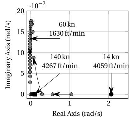
(d) Evolution of the phugoid in autorotation.
