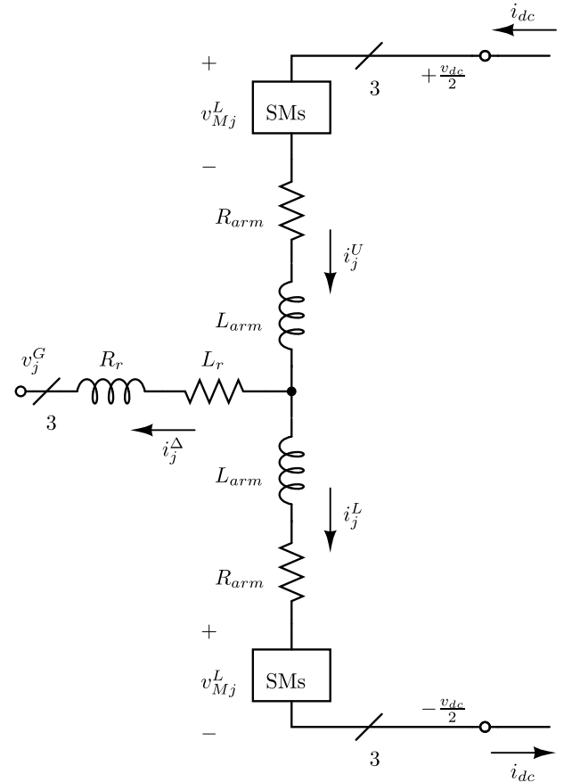
Fig. 1. MMC diagram.
