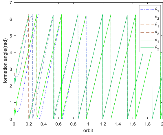
Fig. 7. Formation angles.
