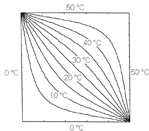
Figuur 3.8. Temperatuurcontouren van het geleidende vierkant in stationaire toestand, met twee randen op 0 °C en twee op 50 °C. Aantal cellen: 50·50.
