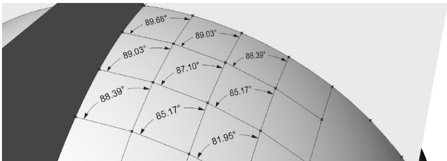
(d) sphere R = 1.20 m; angle 81.95^\circ
