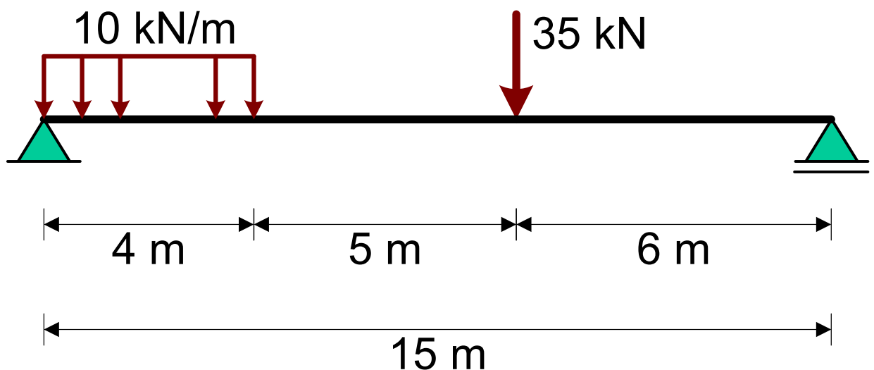
Fig. 1 Voorbeeld constructie
