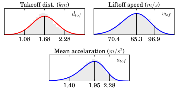
Fig. 9. Take-off parameters
