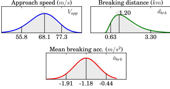
Fig. 15. Landing parameters
