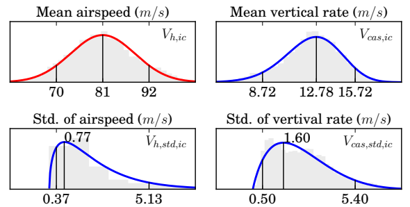
Fig. 10. Initial climb parameters
