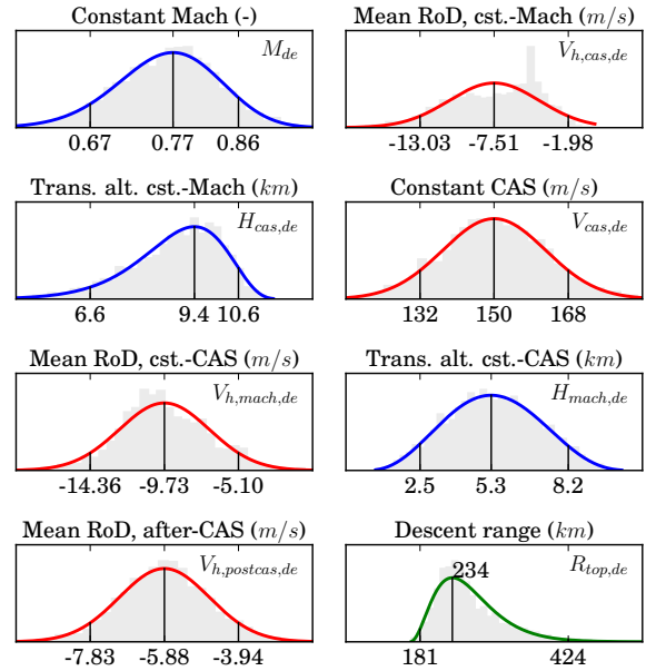
Fig. 13. Descent parameters
