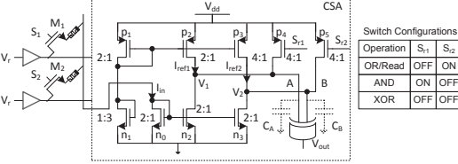
Fig. 5: Current-based SA
