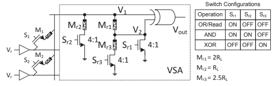
Fig. 6: Voltage-based SA
