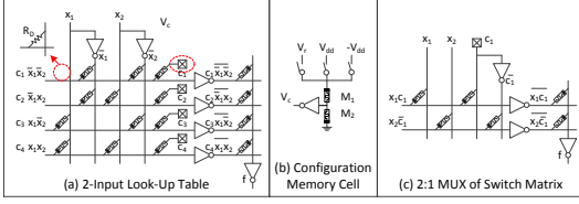
Fig. 5: MFPGA
