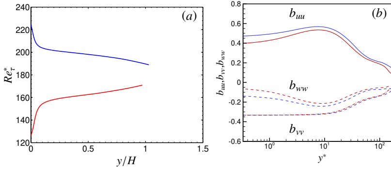
Figure 4.11: Re_\tau^* and anisotropies as a function of y^* for SCCTP. (—) b_{uu} ; (---) b_{vv} ; (---) b_{wv} ; (—) Cold Side; (—) Hot Side.
