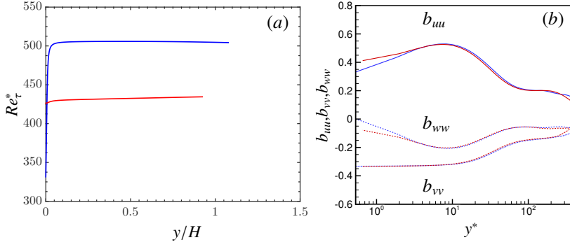
Figure 4.10: Re_\tau^* and anisotropies as a function of y^* for HSC 2 . (—) b_{uu} ; (---) b_{vv} ; (---) b_{wv} ; (—) Cold Side; (—) Hot Side.
