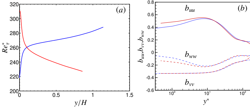
Figure 4.7: Re_{\tau}^* and anisotropies as a function of y^* for LSC 1 . (—) b_{uu} ; (—) b_{vv} ; (---) b_{wv} ; (—) Cold Side; (—) Hot Side.
