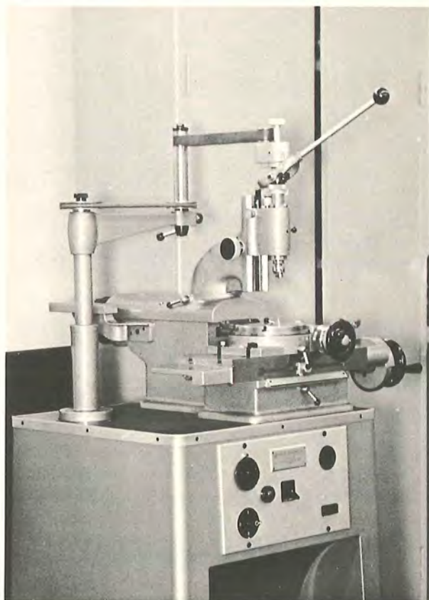
Foto 2 Pointilleermachine
