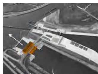
ILLUSTRATIE 4.12 Boezemgemaal Helsdeur.
