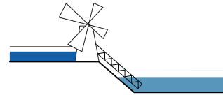
ILLUSTRATIE 3.26 Molen met vijzel: door de uitvinding van de diagonaal geplaatste schroefvijzel kon vanaf 1630 een hoogteverschil van meer dan 1,50 meter overbrugd worden. De vijzel werd eerst van hout gemaakt en later van staal.
