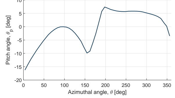
(d) Max C_P - Pitch schedule
