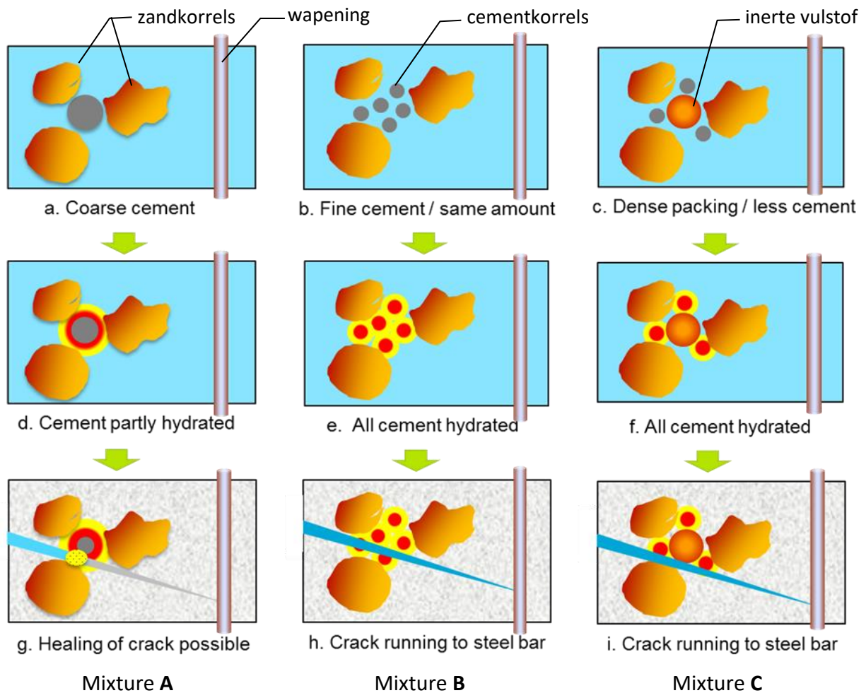
Fig. 9 Karakteristieken van betonmengsels. A) Mengsel met grof cement; B) Mengsel met fijn cement; C) Fijn cement met dichte korrelepakking van toeslagmateriaal en en/of inerte vulstof (bijvoorbeeld zeer fijn zand). (● cement; ● inner product; ● outer product; ► scheur)
